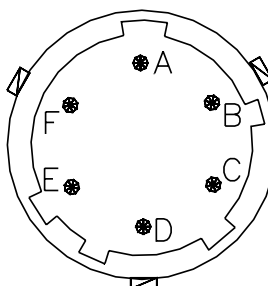
Connecteur 6 broches VPT07RA10-6PT2 (PT02A-10-6P)
