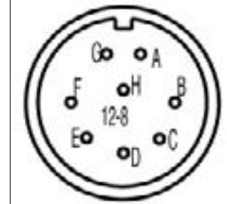
Connecteur 8 broches PC02E-12-8P Bendix
