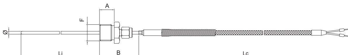
TC1M B: Avec raccord à compression coulissant
