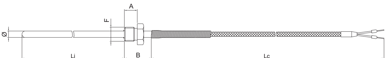
TC1 C: Mit festem Anschluss
