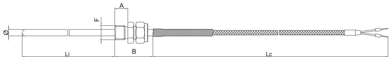
TC1 B: Mit einstellbarer Klemmverschraubung
