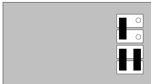
Collegamento 4 fili Anschluss 4-Leiter Connection 4 wire Conexión 4 hilos Connexion 4 fils Ligação 4 fios
