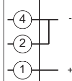
Carte ALIMENTATION CAPTEUR
