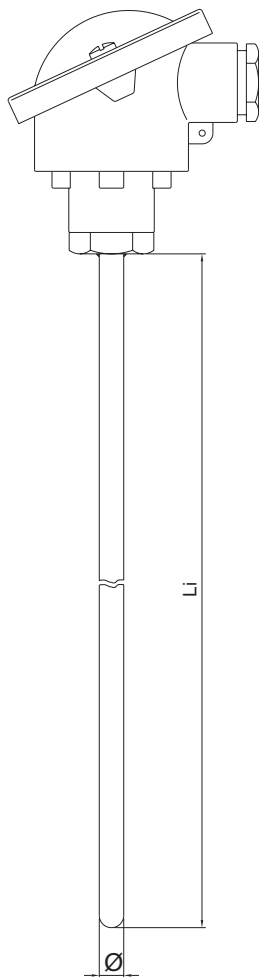
TR6M A senza raccordo
