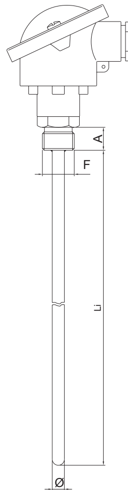
TR6M D con raccordo saldato sottotesta
