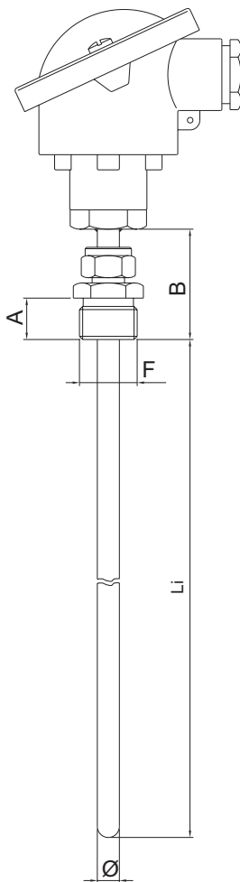
TR6M B con raccordo a compressione scorrevole
